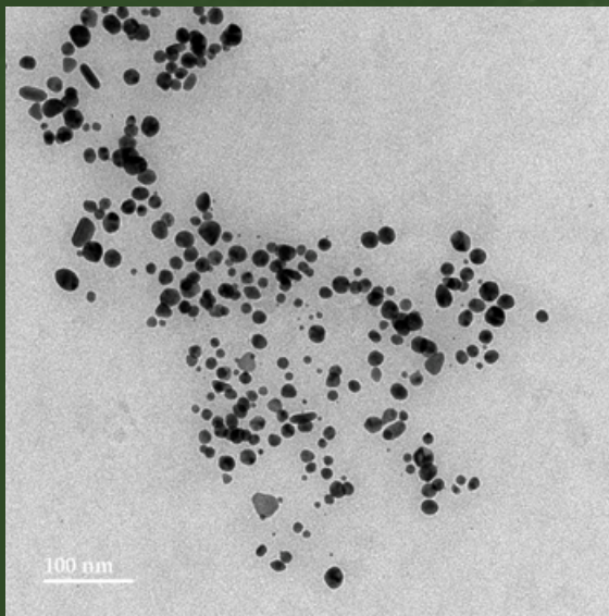
TEM Image of LKP-AU-00178
